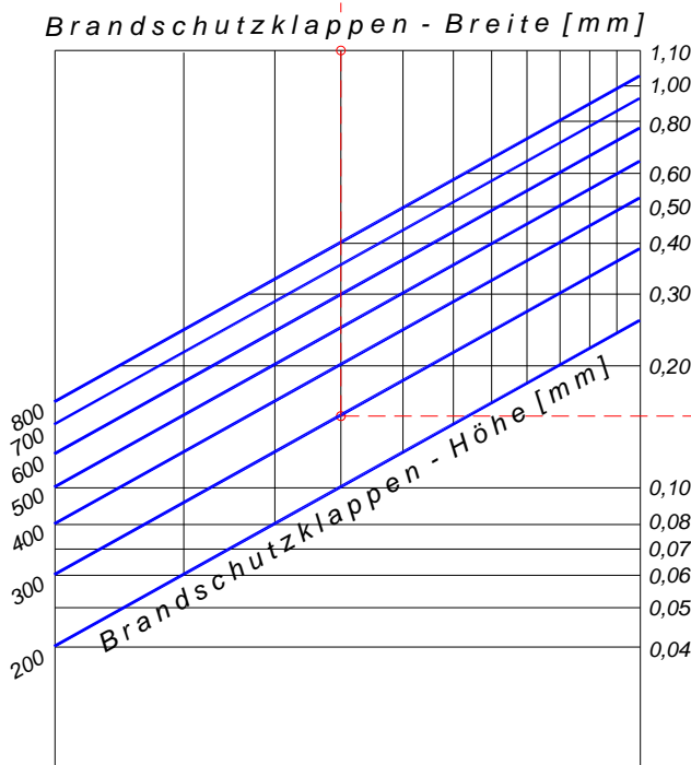
Brandschutzklappen - Breite [mm]
